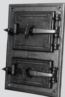
DOOR 1. 13''w x 19''h
